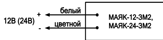
Рис.1. Схема подключения.
