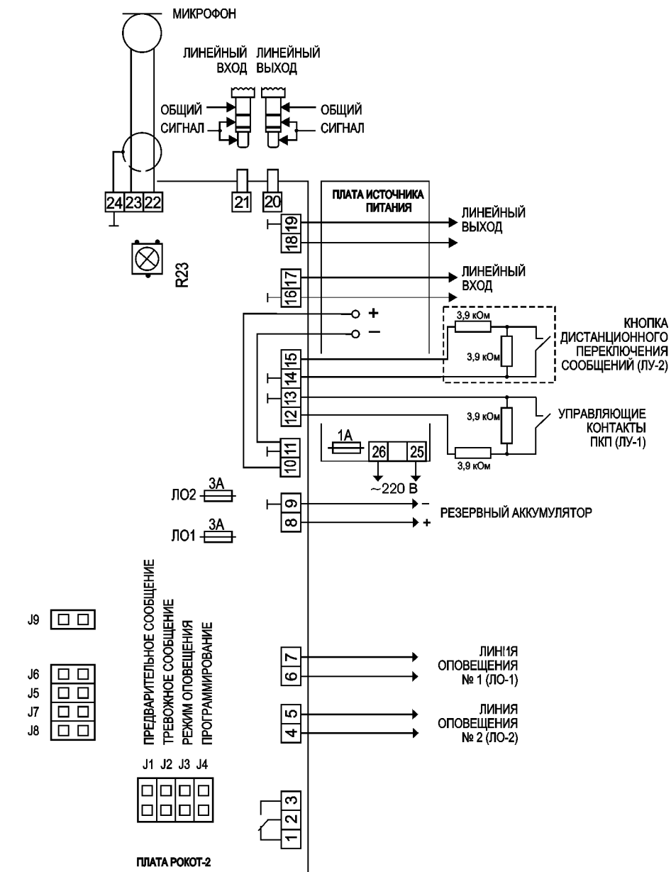
Рис. 2 Схема подключения «РОКОТ-2»
