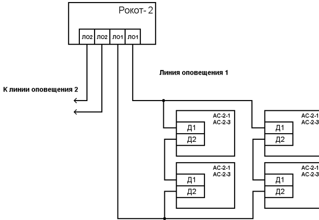
Рис. 4 Подключение акустических систем АС-2-1, АС-2-3 (со встроенной схемой контроля исправности линий оповещения)
