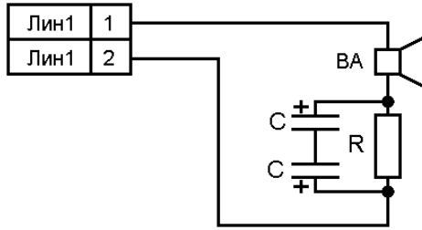
Рис. 3 Схема электрическая «АС-2-1»
