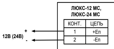
Рис.1. Схема подключения.
