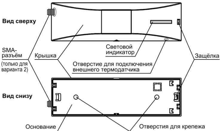
Рис.1 Конструкция сигнализатора. Вид сверху и снизу
