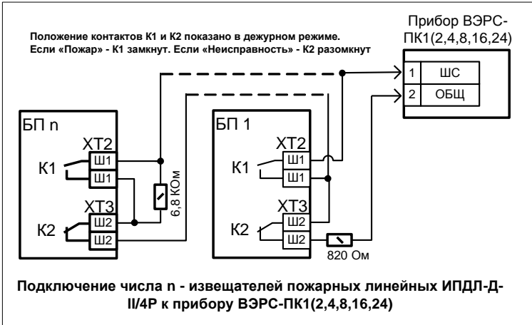
Рисунок Б5. Схема включения линейных дымовых извещателей ИПДЛ-Д-II/4P.
