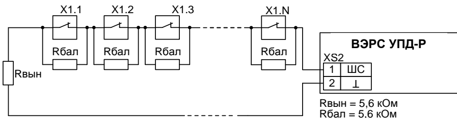
Рисунок 10 Схемы подключения ШС к пожарному типу устройства «ВЭРС УПД-Р»
