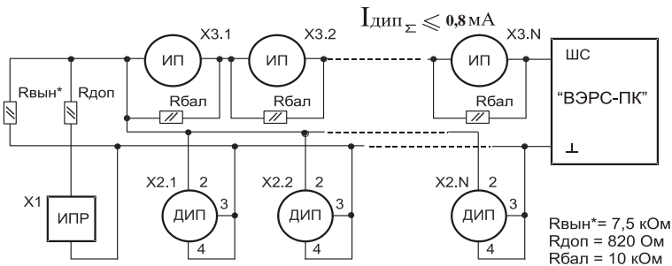
Рисунок.Б4. Комбинированная схема включения ШС. Однопороговый алгоритм с верификацией.
