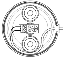
Рисунок 5 – Монтаж провода в основании датчика
