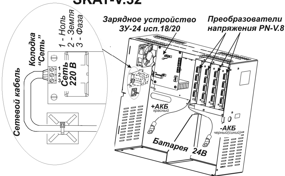
Рисунок 1 - Внешний вид блока с открытой крышкой и подключение сетевых проводов и провода заземления
