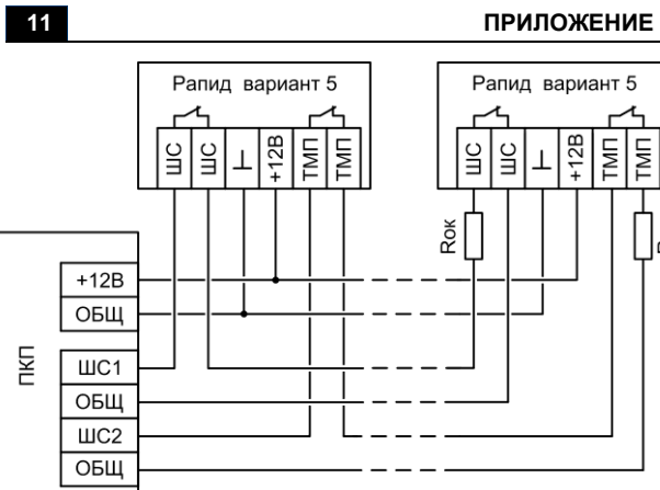
Рис.2 Схема подключения извещателя к ПКП
