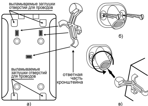
Рис.1 а) Вид на заднюю стенку извещателя. б) Крепление кронштейна (основания). в) Схема соединения кронштейна и держателя
