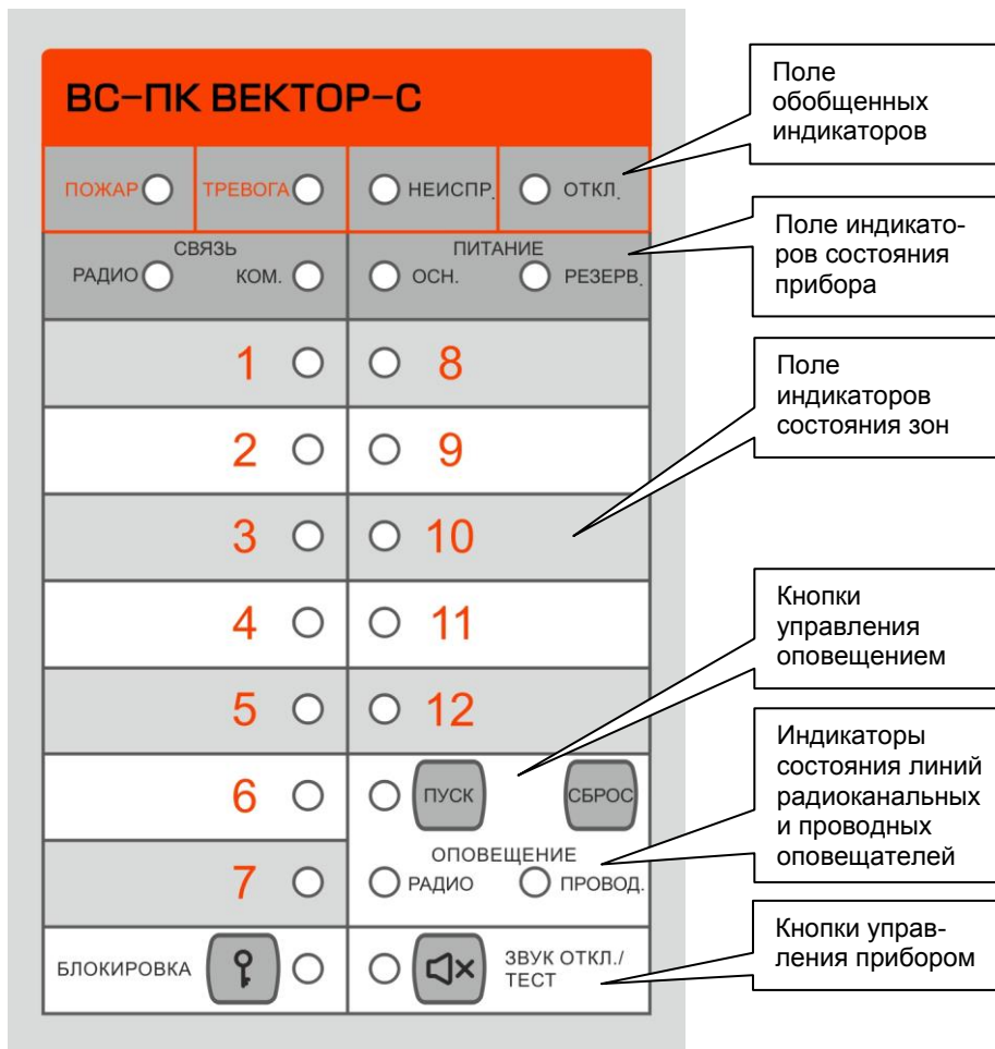
Рис.1. Внешний вид панели индикации и управления прибора.
