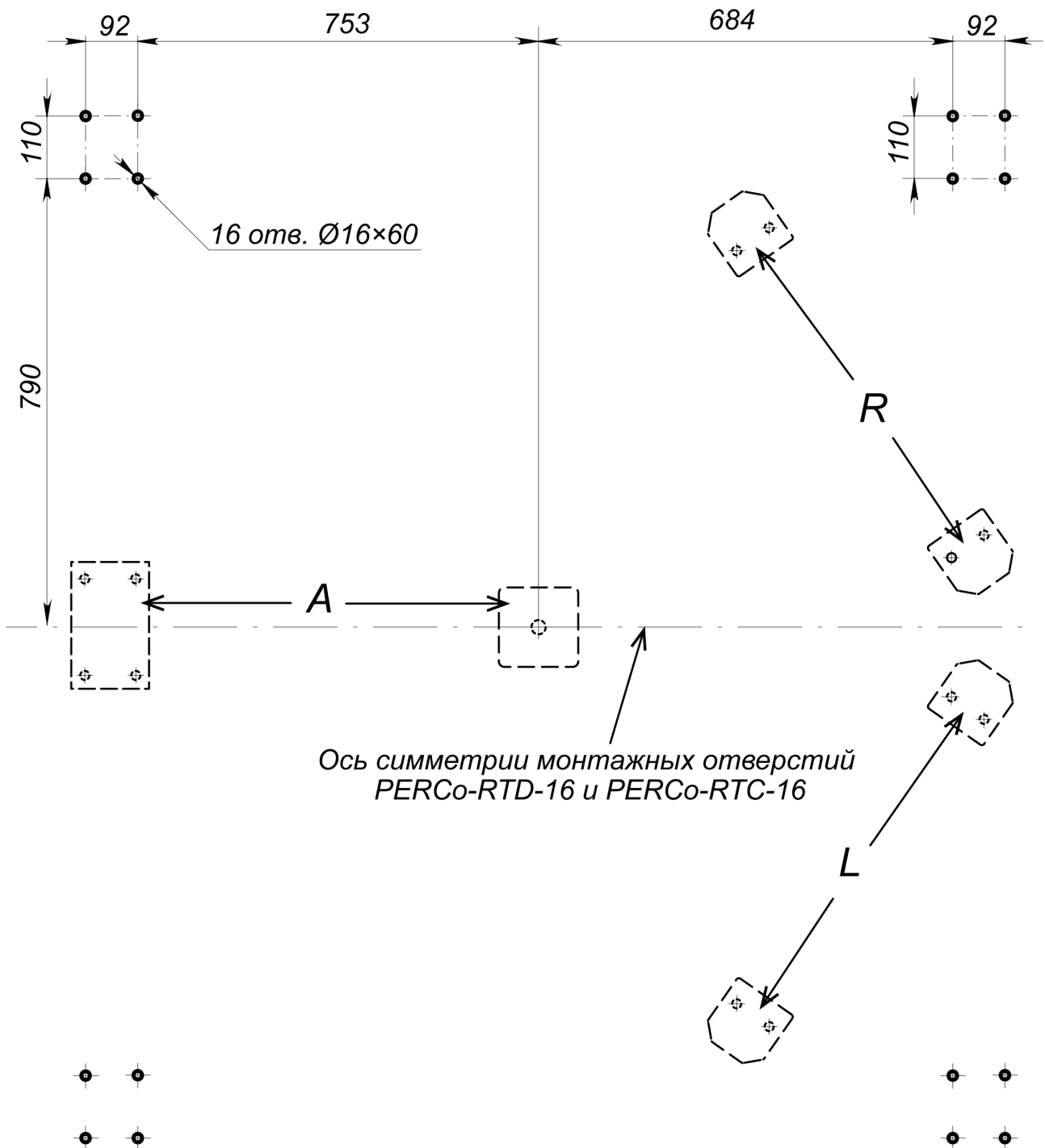
Рисунок 3. Схема разметки отверстий для установки крыши PERCo-RTC-16
