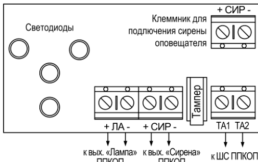
Рис.1 Схема подключения оповещателя к ППКОП
