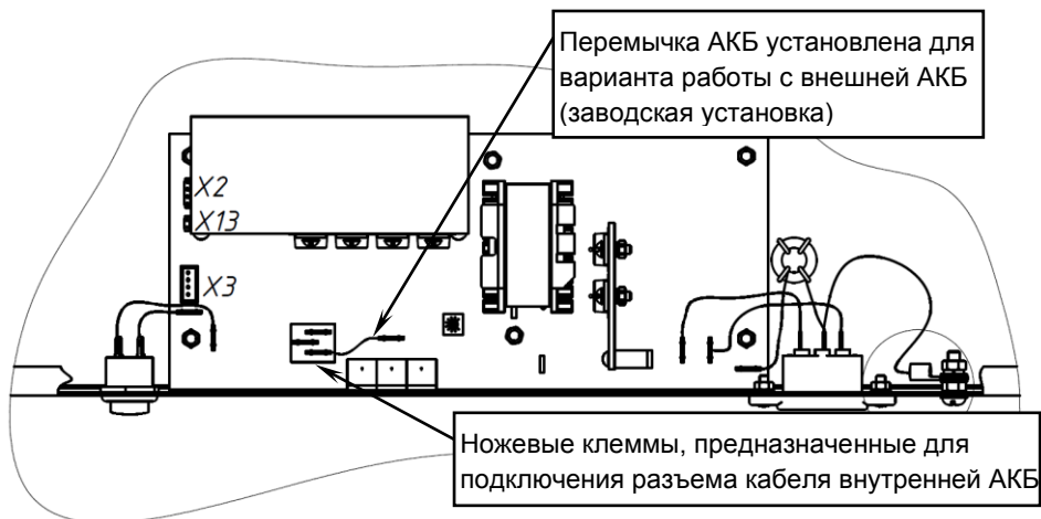
Рисунок 3 – вид на плату изделия
