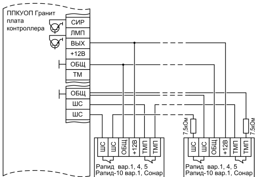
Рис.А3 Схема подключения охранных извещателей Рapid вар.1,4,5, Рapid-10 вар.1, Сонар (тампер извещателя подключён к отдельному ШС)
