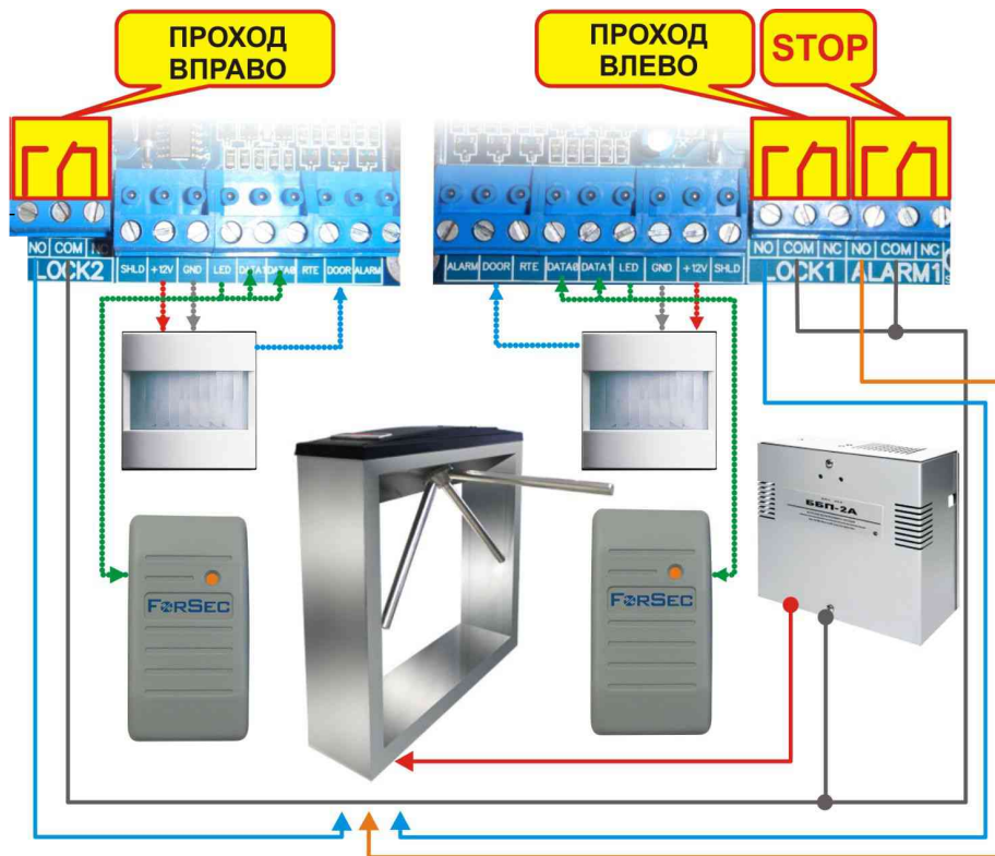
Рисунок 12: Управление турникетом
