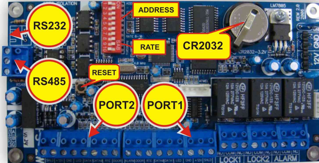
Рисунок 3: Плата контроллера FS-2W
