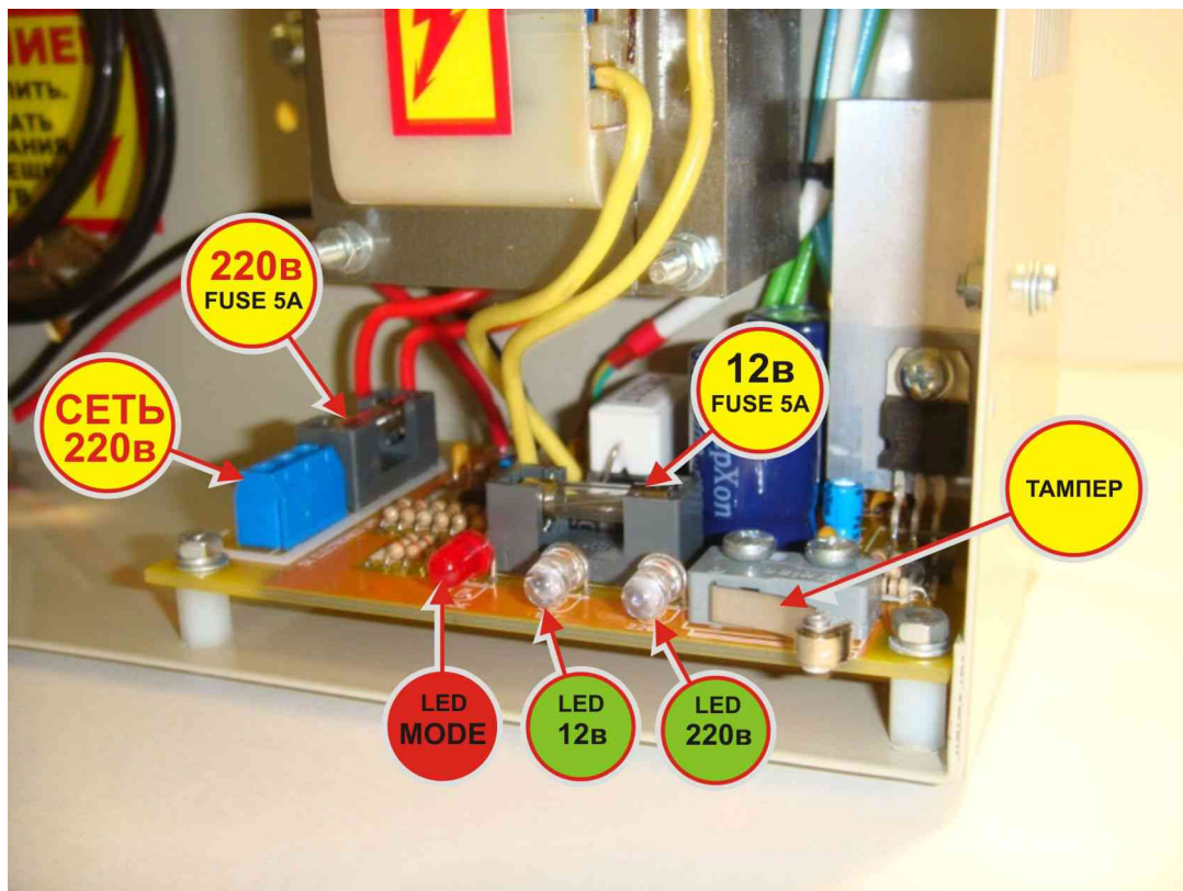
Рисунок 2: Источник питания
