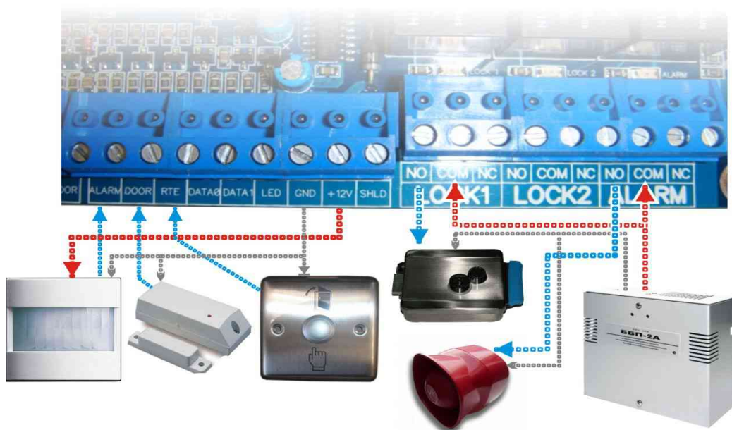
Рисунок 7: Подключение внешних устройств
