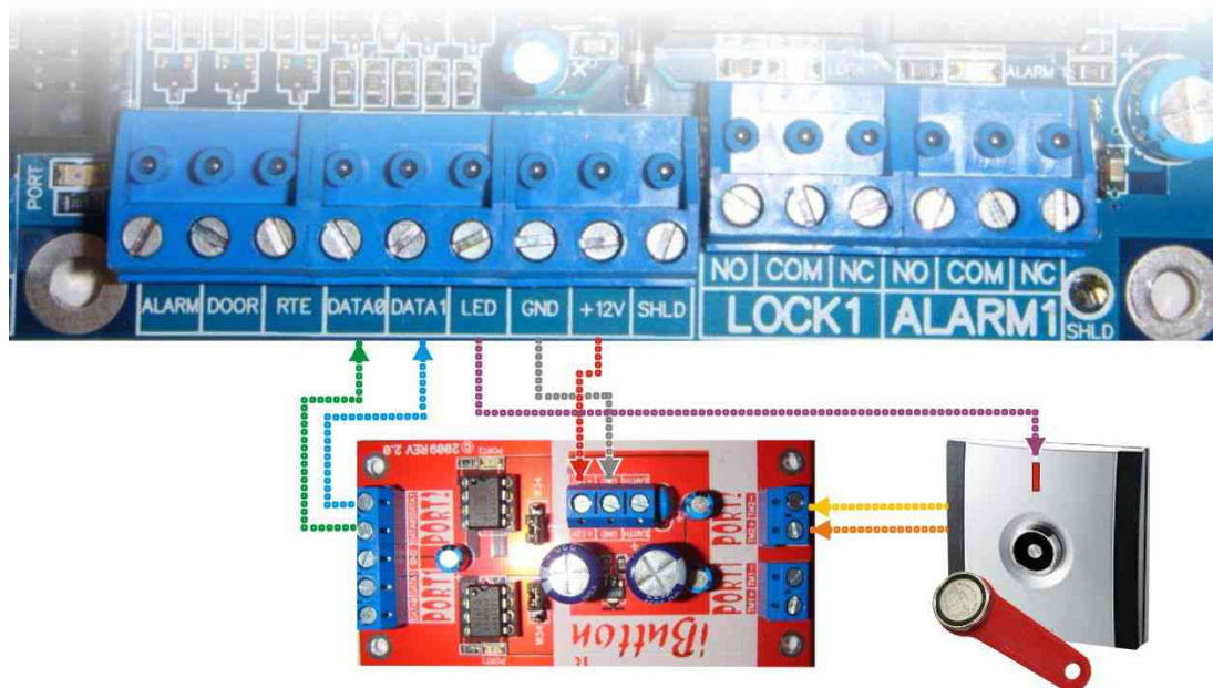
Рисунок 8: Подключение преобразователя интерфейса FS-WT
