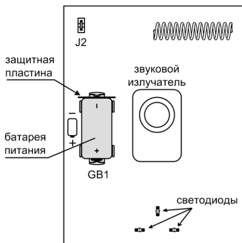
Рис.4 Плата сирены
