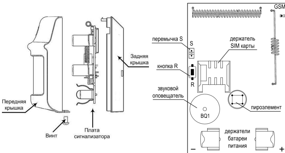
Рис.1 Конструкция сигнализатора
