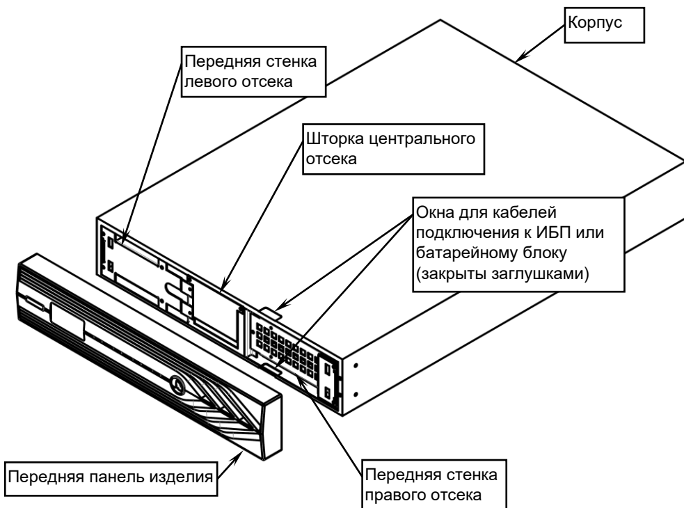
Рисунок 1 – Общий вид изделия со снятой передней панелью
