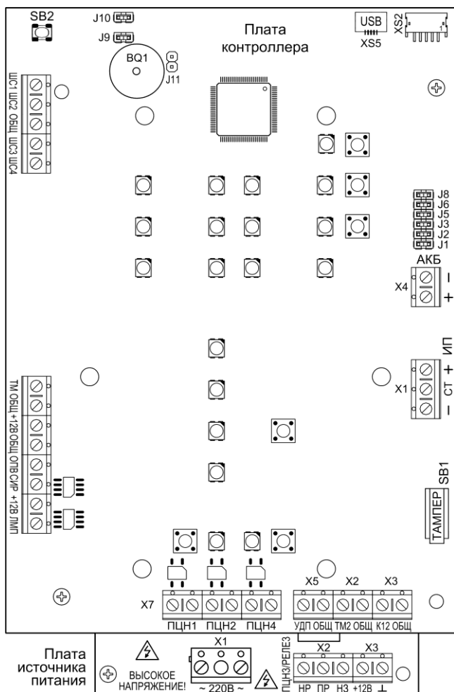
Рис.1 Плата контроллера Гранит-4 (вид со снятой панелью индикации и управления) и плата источника питания (видимая часть)
