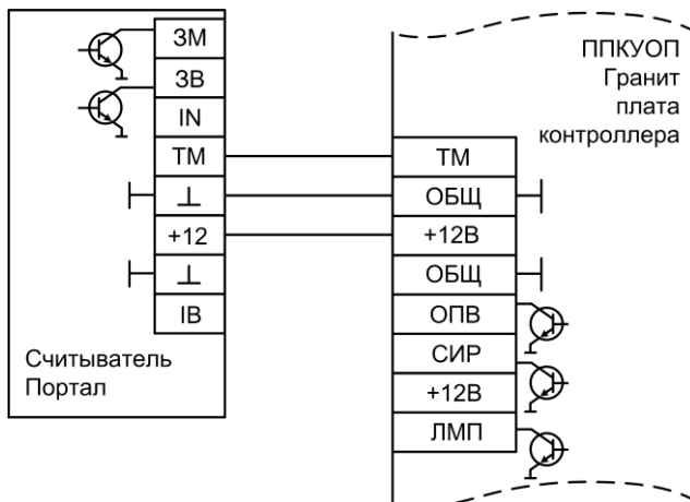
Рис.57 Схема подключения счетывателя «Портал»
