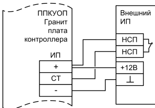
Рис.58 Схема подключения внешнего источника электропитания (ИП)
