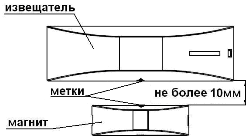
Рис.11 Общий вид извещателя ПОЛЮС-Р2
