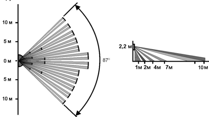
Рис.8 Диаграмма зоны обнаружения
