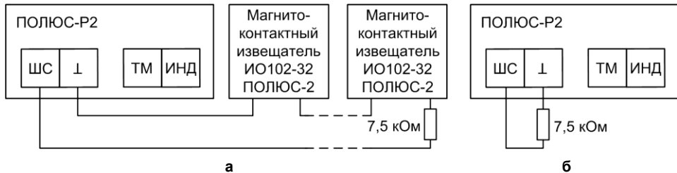
Рис.12 Схема подключения извещателя
