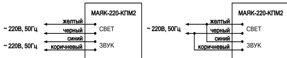
Рис.1. Схема подключения.
