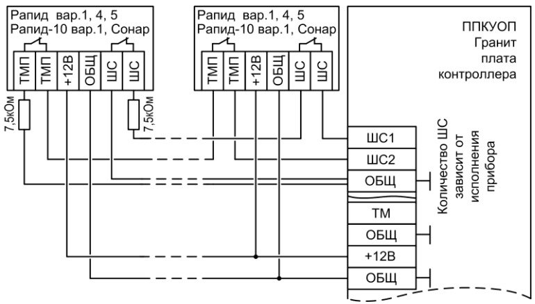
Рис.Б5 Схема подключения охранных извещателей Rapid вар.1,4,5, Rapид-10 вар.1, Сонар (тампер подключён к отдельному ШС)
