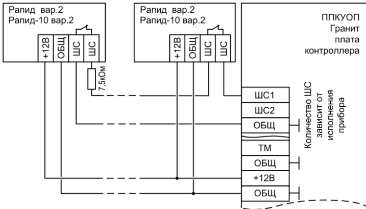
Рис.Б6 Схема подключения охранных извещателей Rapid вар.2, Rapid-10 вар.2
