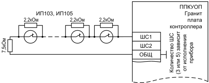
Рис.Б3 Схема подключения пожарных электроконтактных извещателей
