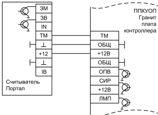
Рис.Б7 Схема подключения считывателя «Портал»
