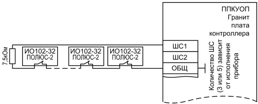
Рис.Б4 Схема подключения охранных магнитоконтактных извещателей
