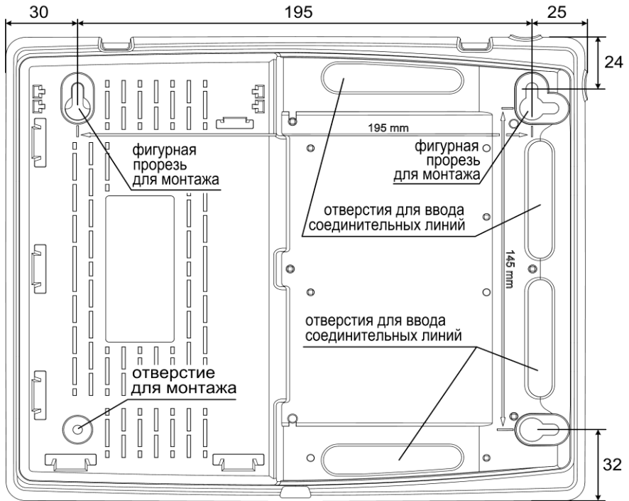
Рис.3 Задняя стенка прибора. Присоединительные размеры
