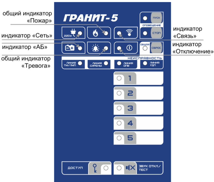
Рис.2 Панель индикации и управления прибора Гранит-5-48В
