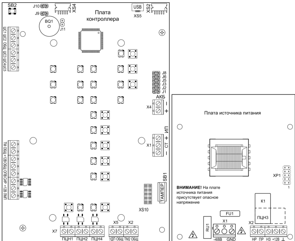
Рис.1 Плата контроллера Гранит-5-48В (вид со снятой панелью индикации и управления) и плата источника питания (плата контроллера снята с платы источника питания)
