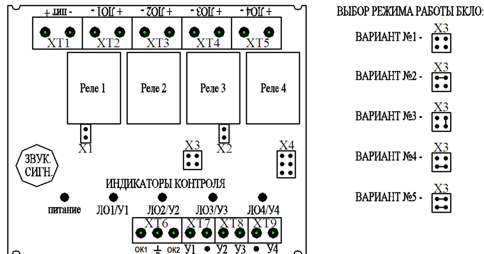
Рисунок-2 Схема клемм подключения и выбора варианта включения БКЛО
